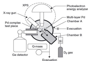
Fig.5 Iwamura’s Gas Diffusion Apparatus
