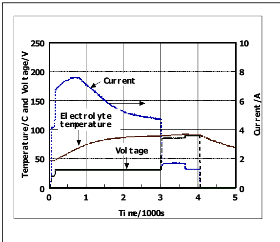
Fig. 1: Parameter changes for electrolysis.
